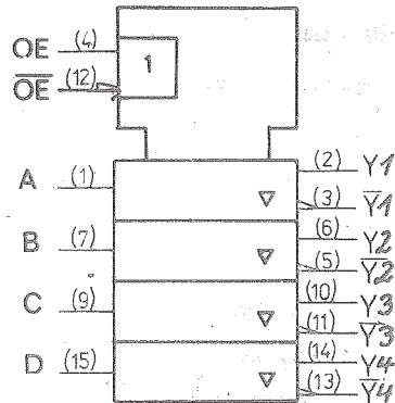
Bild 2: Schaltungskurzzeichen und Anschlußbelegung
